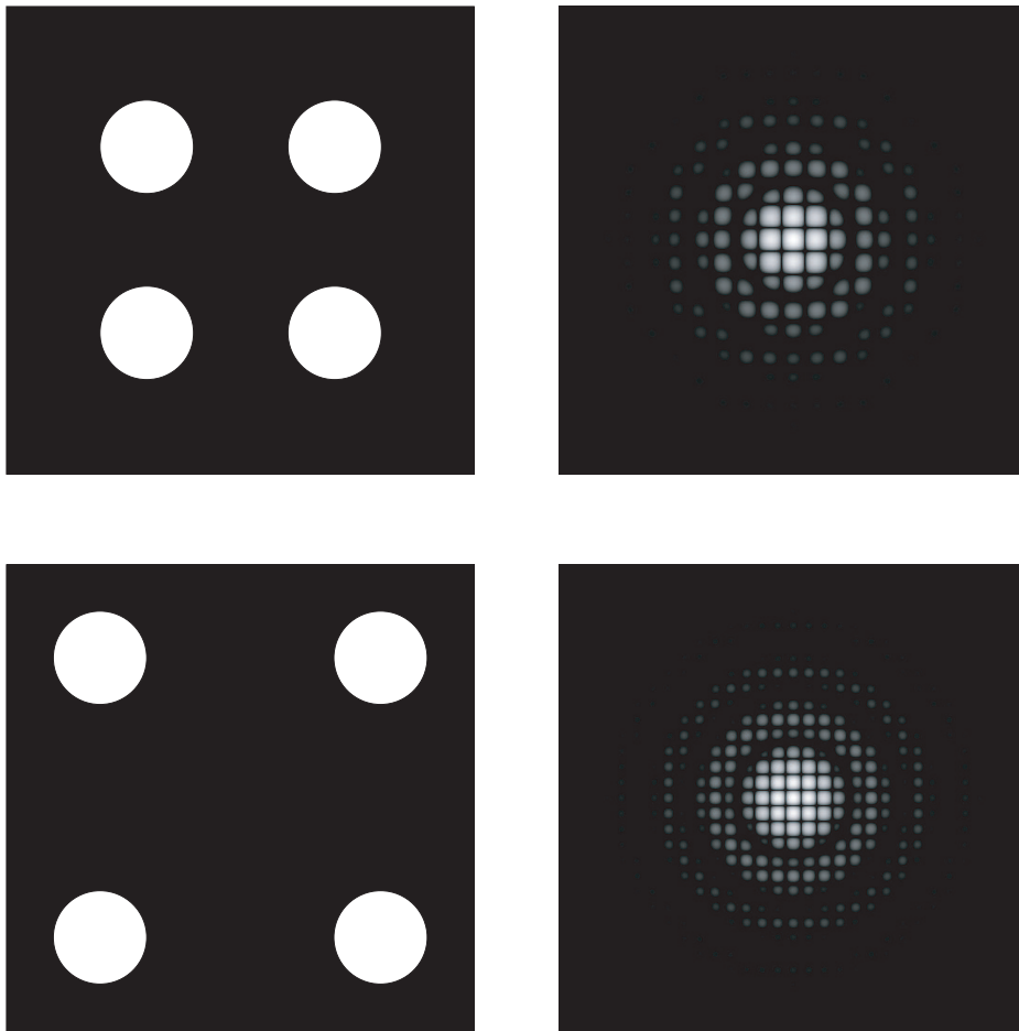
Abbildung 3: Vierlochblenden (links) und erzeugte Beugungsbilder (rechts). Das Verhältnis von Lochdurchmesser : Lochabstand ist oben 1:2, unten 1:3.
